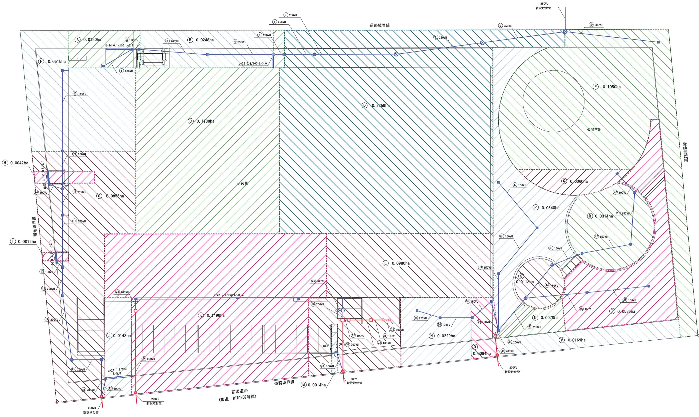
排水区画割平面図 S=1/200
