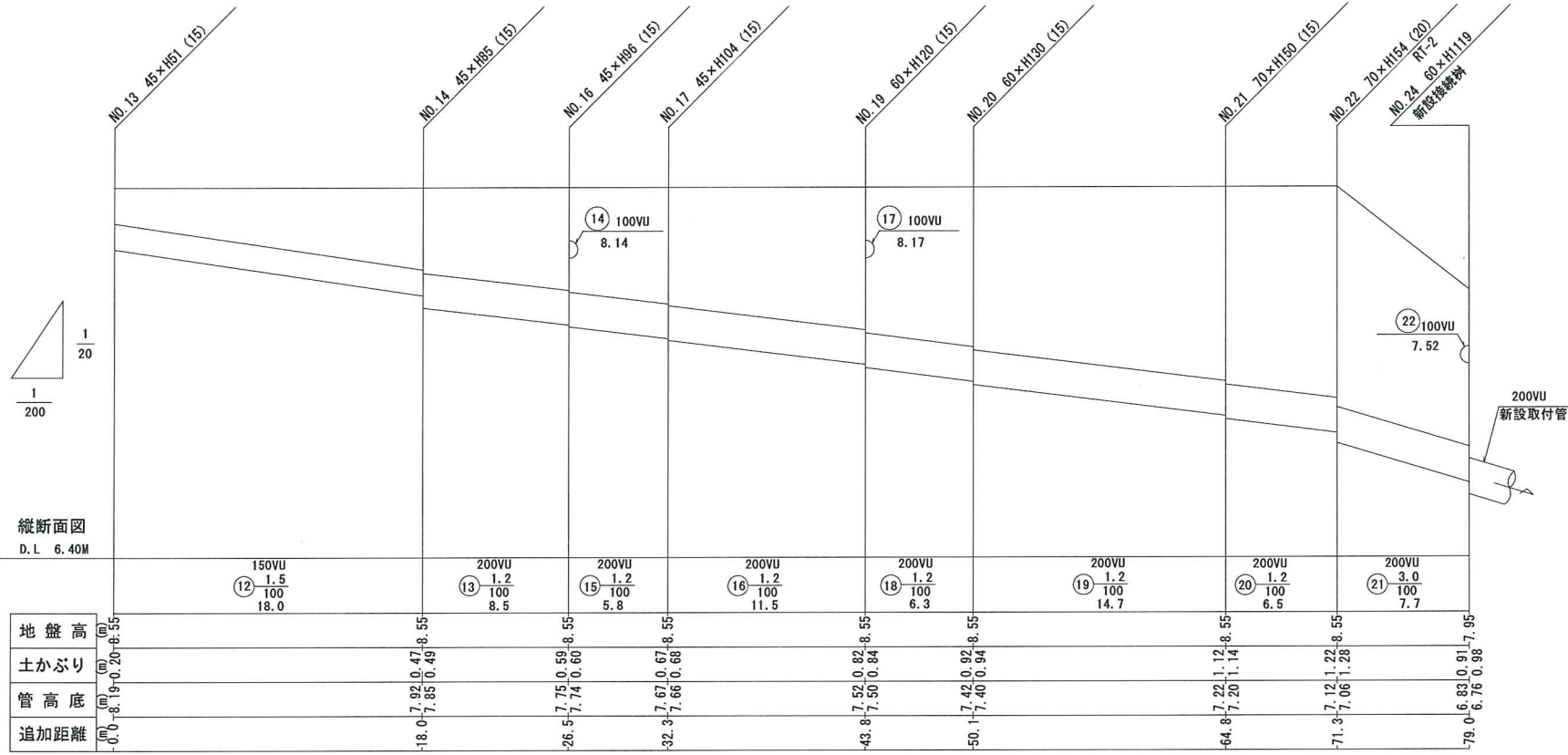
縦断面図
